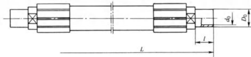
图 2 卡套式液压软管总成
