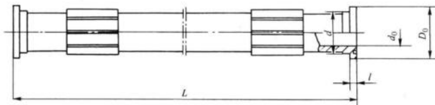
图4 法兰式液压软管总成
