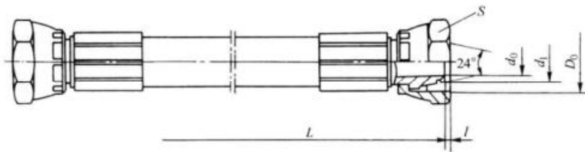
图5 24° 锥密封式液压软管总成
