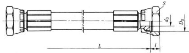
图3 焊接式或快换式液压软管总成
