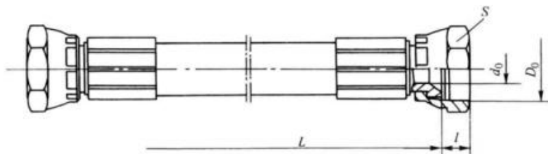
图 1 扩口式液压软管总成
